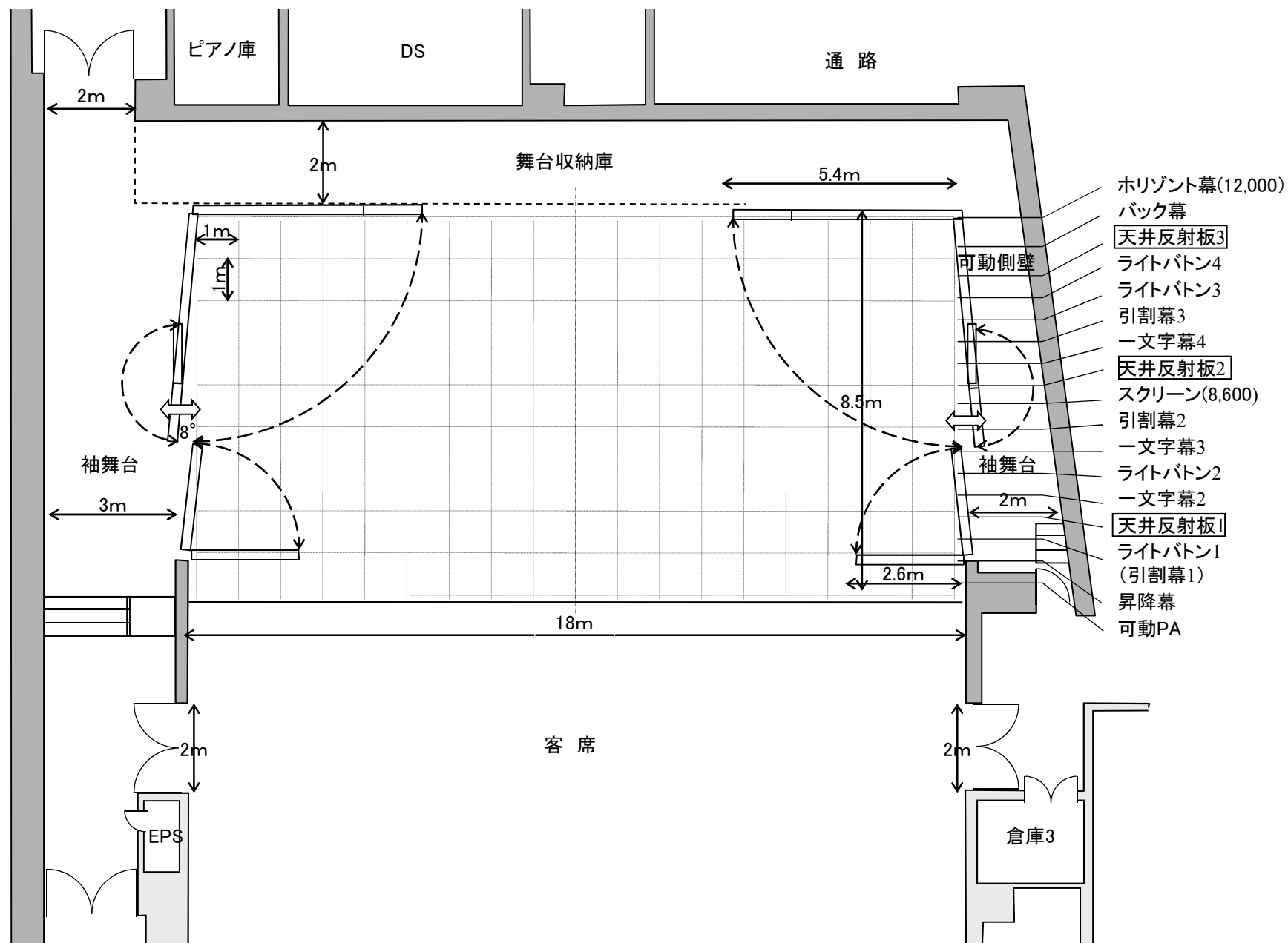
ふれあいホール舞台平面図
