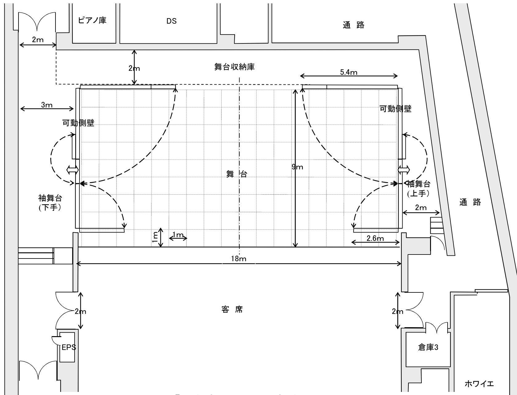
「ふれあいホール」舞台平面図
