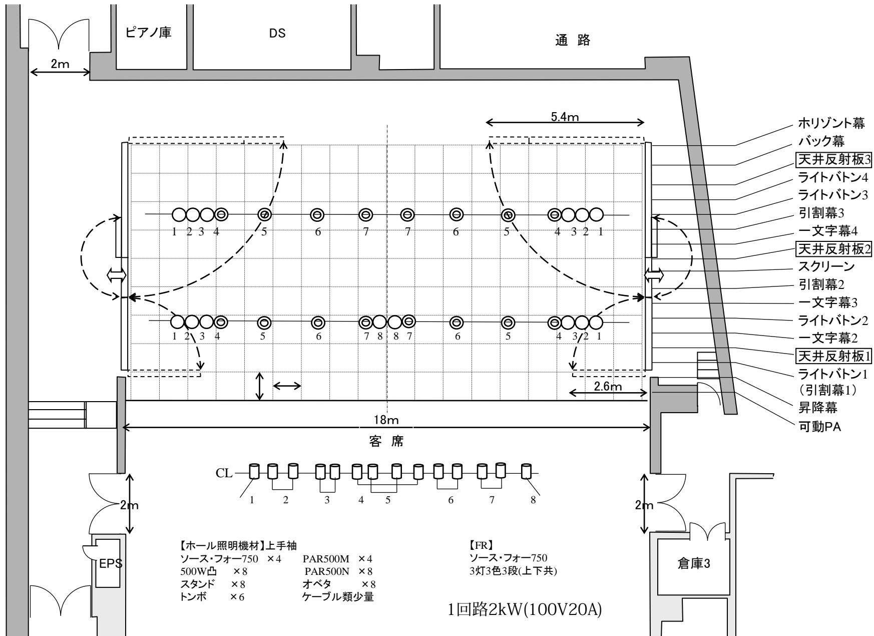
ふれあいホール舞台照明設備平面図
