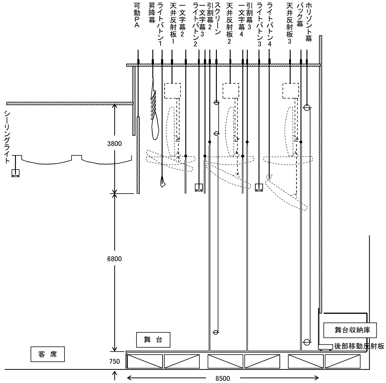
ふれあいホール舞台断面図
